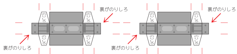
パンタA
