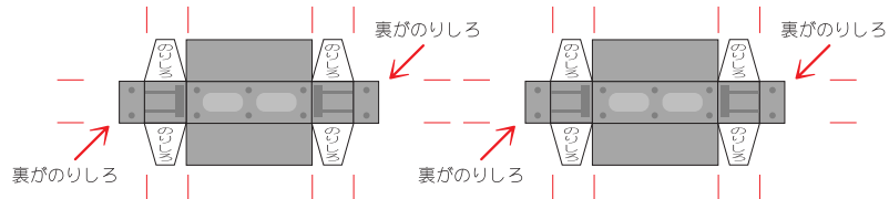
パンタA
