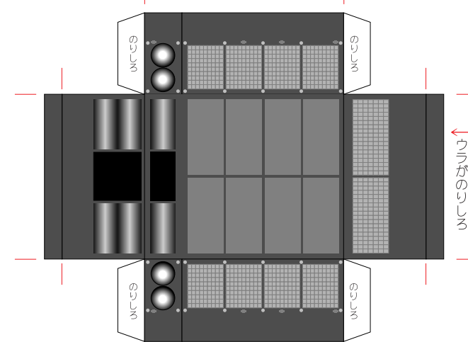
床下機器
